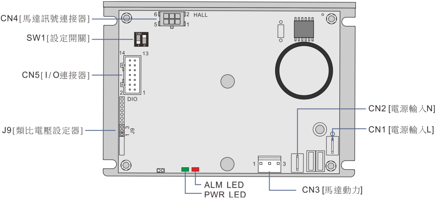
Fig 2 連接器與面板功能
