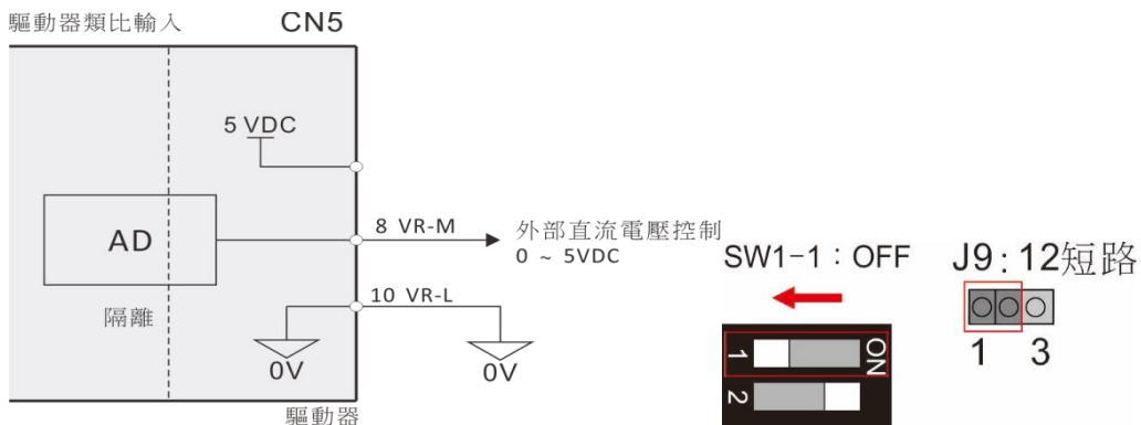
Fig 13 類比輸入使用外部電壓 0 – 5 VDC
