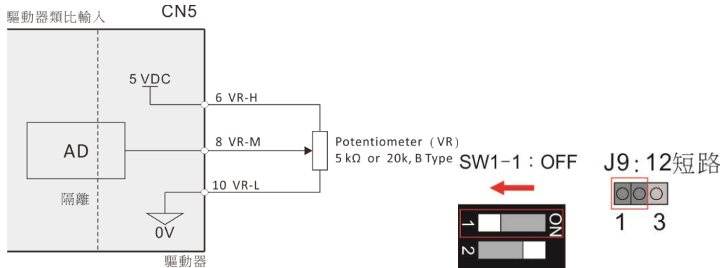
Fig 12 類比輸入使用外部電位器(VR)
