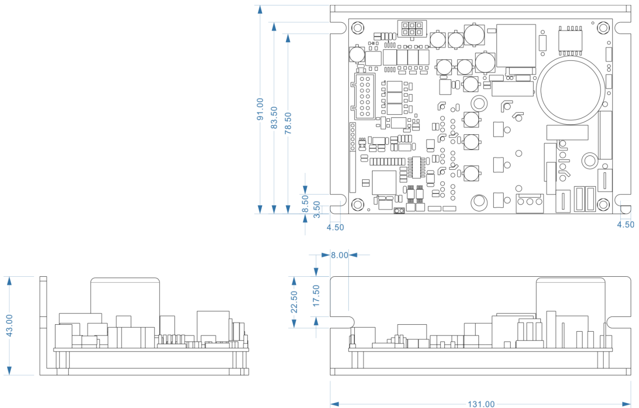
Fig 18 ASDS-A200□□ / ASDS-B200□□ 安裝尺寸圖
