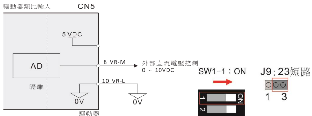
Fig 14 類比輸入使用外部電壓 0 – 10 VDC
