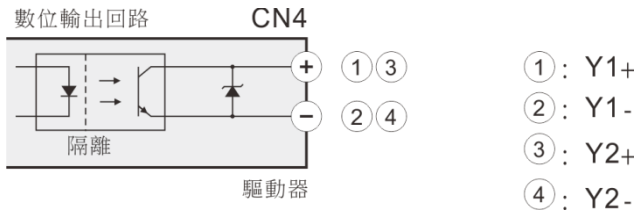
Fig 9 數位輸出內部回路
