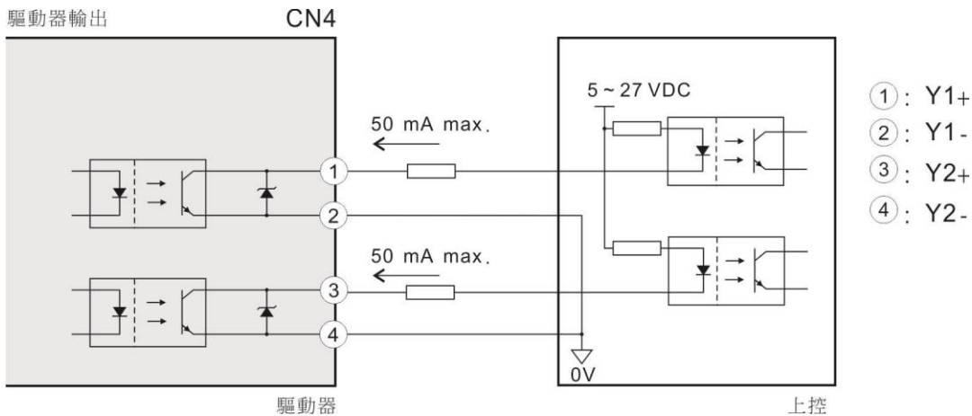
Fig 10 數位輸出外部裝置(上控)SINK 的連接
